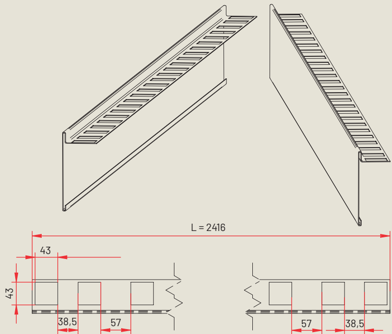
Angolo interno Internal corner
