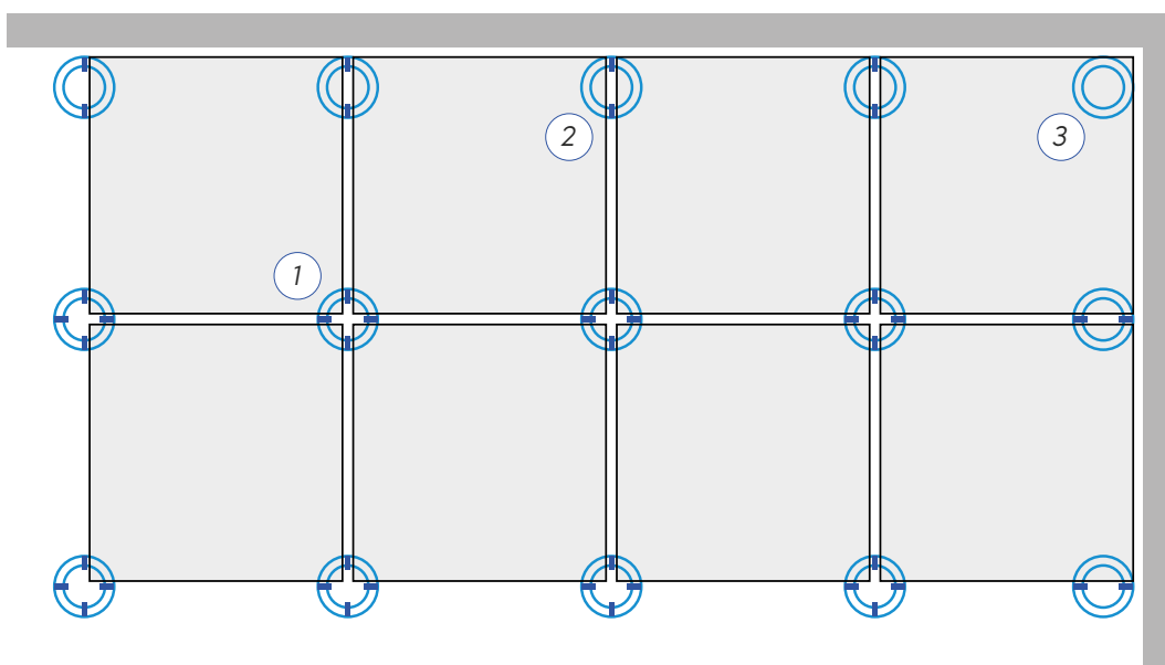
Centre plancher Mitte des Doppelbodens
