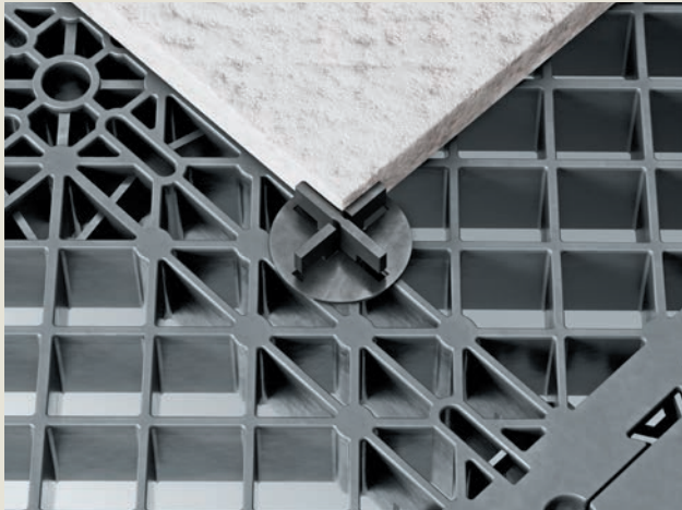
Beispiele für die Positionierung von Platten mit DM..
