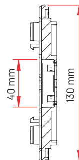
Version non basculante pour plots NM
