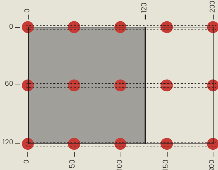
Dalles | Format 120 x 120 cm - Entraxe lambourde | Schienenabstand 60 cm
