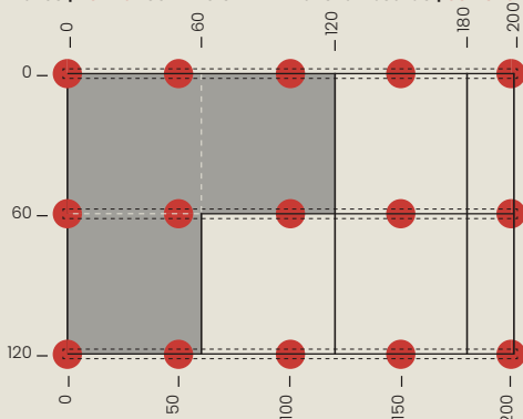
Dalles | Format 40 x 60 cm - Entraxe lambourde | Schienenabstand 60 cm
