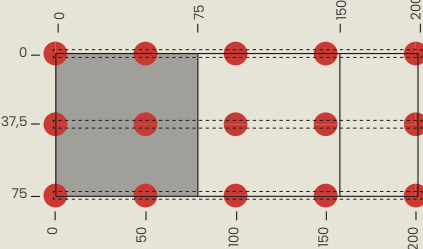
Dalles | Format 80 x 80 cm - Entraxe lambourde | Schienenabstand 40 cm
