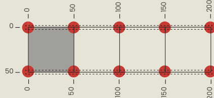
Dalles | Format 60 x 60 cm - Entraxe lambourde | Schienenabstand 60 cm
