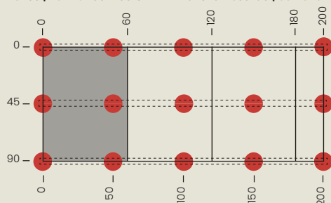
Dalles | Format 60 x 90 cm - Entraxe lambourde | Schienenabstand 45 cm
