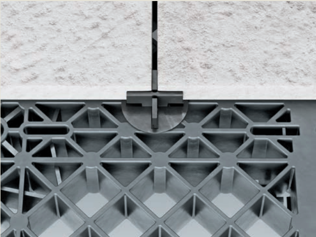
Exemples de positionnement des dalles avec le distanciateur DM.
