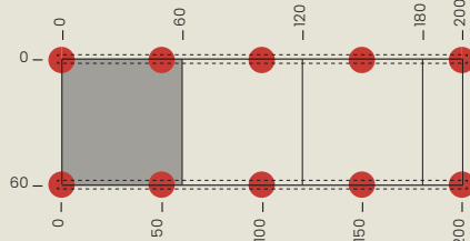
Dalles | Format 75 x 75 cm - Entraxe lambourde | Schienenabstand 37,5 cm
