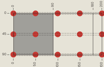
Dalles | Format 90 x 90 cm - Entraxe lambourde | Schienenabstand 45 cm
