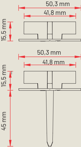
Écarteur Mini DM avec embout pour les fonds en sable et gazon Kreuzfuge Mini DM mit Nagel für Sand- und Rasen
