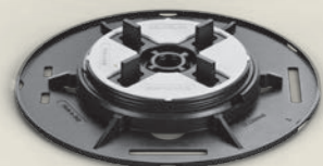
New Maxi NM O dès H 15 mm ab H 15 mm
